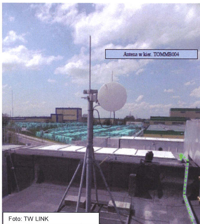
Widok instalacji radiokomunikacyjnej Stacja Netia TOMMB009 - TOMMM00017 Tomaszów Mazowiecki, ul. Włókiennicza 12/18.
